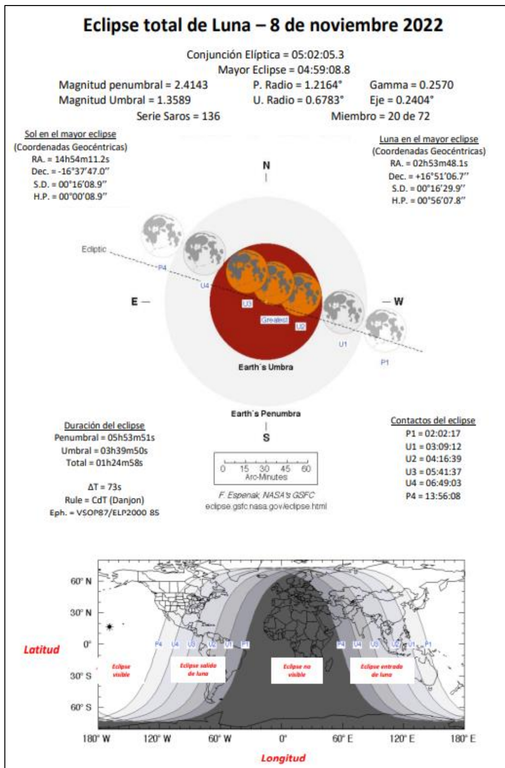
Figura 6. Eclipse total de Luna.
