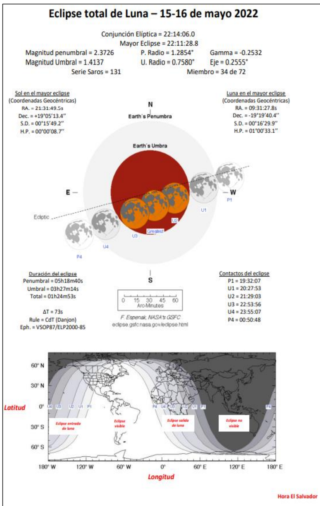
Figura 4. Eclipse total de Luna.
