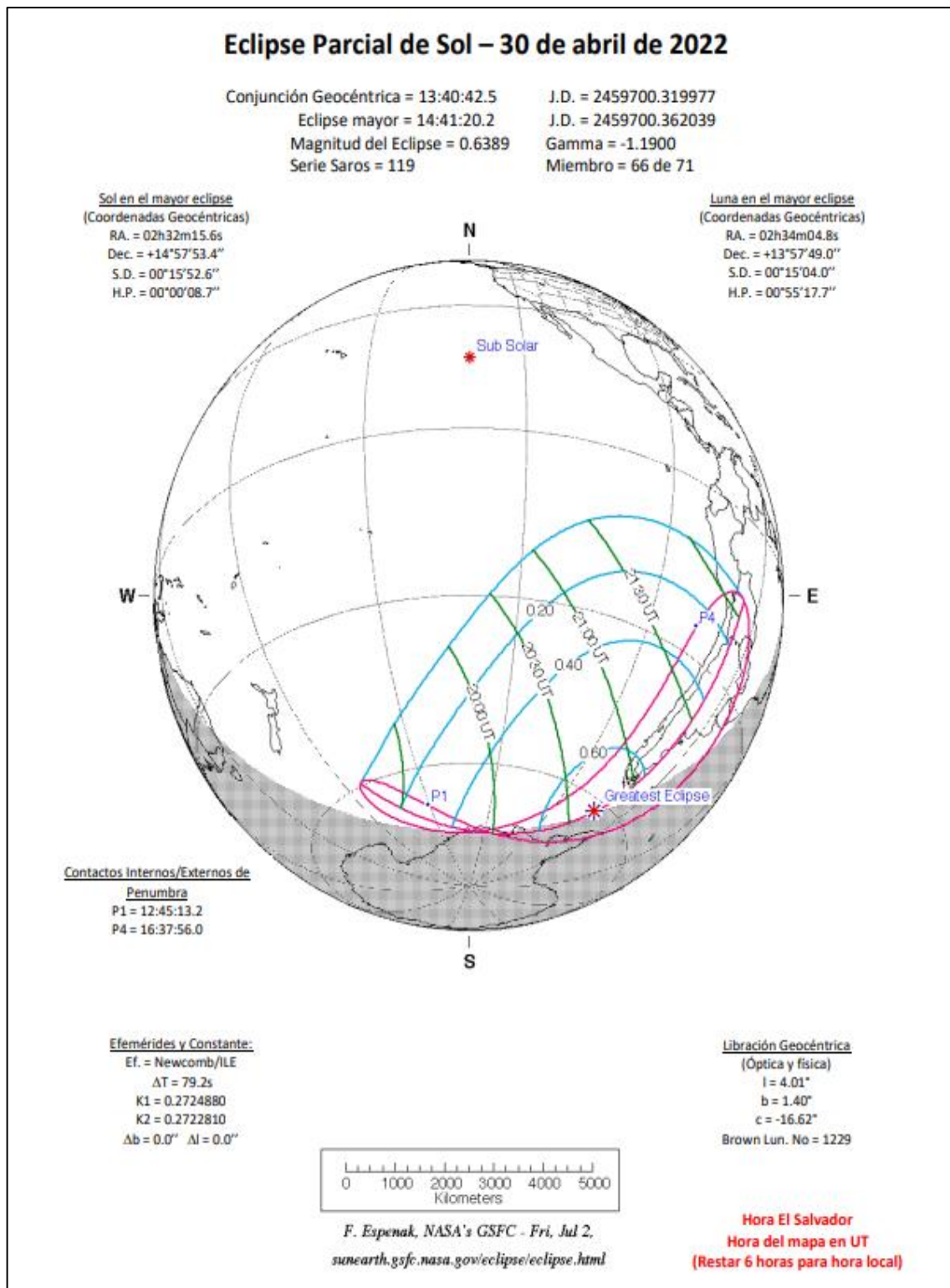
Figura 3. Eclipse Parcial de Sol Fuente: MARN con datos retomados de The Astronomical Almanac for the year 2022.
