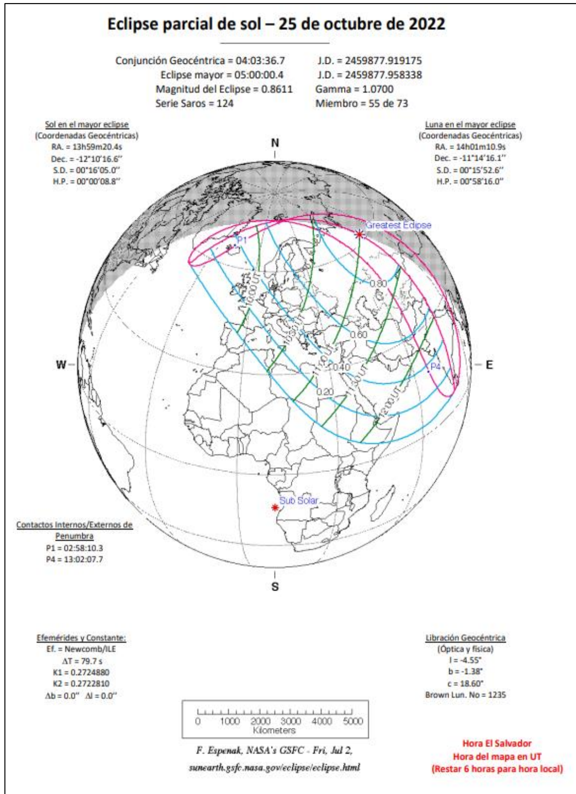
Figura 5. Eclipse parcial de Sol.
