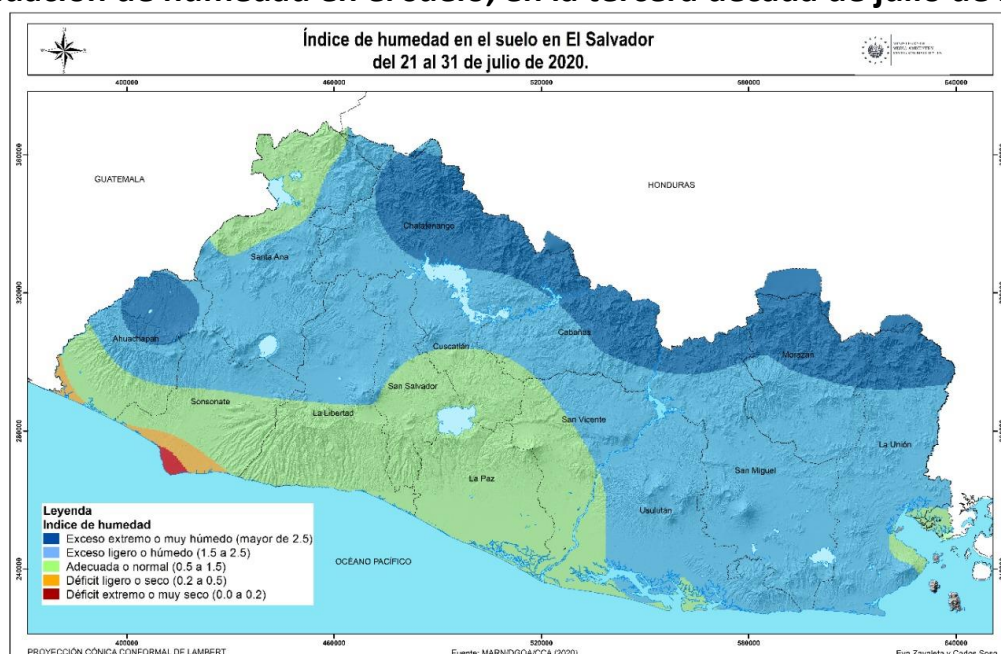
Figura 3. Mapa de Índice de humedad en suelo, del 21 al 31 de julio de 2020.
