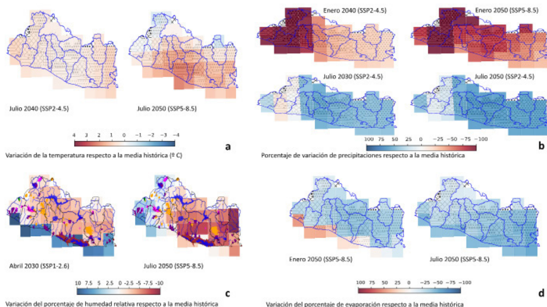
Figura 1. a. Proyecciones de temperatura bajo distintos escenarios de emisiones; b. Proyecciones de precipitación bajo distintos escenarios de emisiones; c. Proyecciones de humedad bajo distintos escenarios de emisiones; d. Proyecciones de evaporación bajo distintos escenarios de emisiones. Fuente: Gauss, 2025a.
